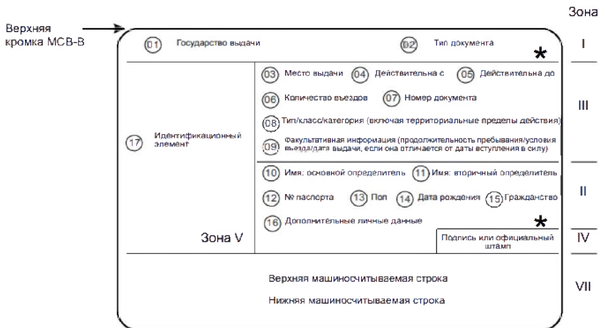
Рисунок 6 – Расположение элементов данных визы формата «В», не в масштабе
