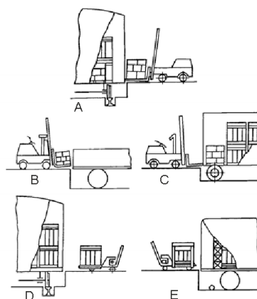
А, В, С – механизированным способом; D, Е – с помощью средств малой механизации Рисунок 4 – Варианты выполнения погрузо-разгрузочных работ с тарно-штучными грузами
