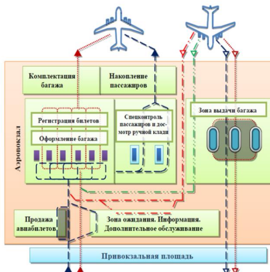
Рисунок 3 – Основные технологические процессы в аэропорту
